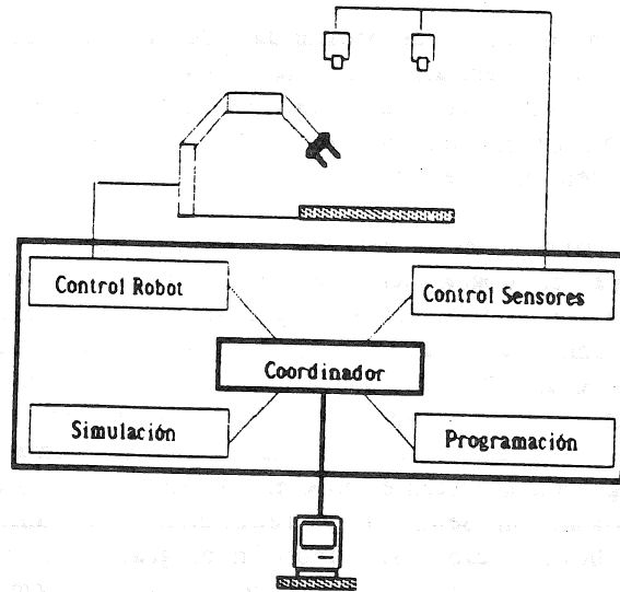
figura 1.- Estructura funcional de MSIM
