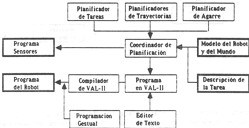
figura 2.- Estructura funcional del módulo de programación
