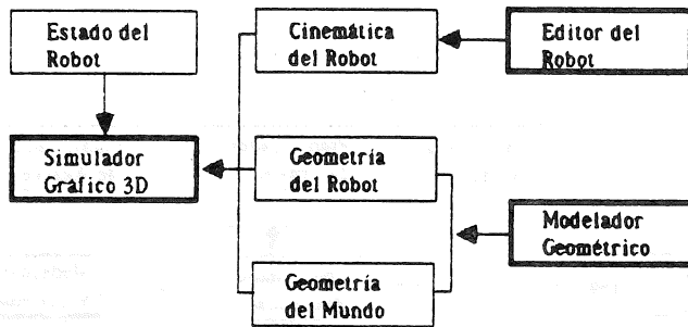
figura 3.- Estructura funcional del módulo de simulación
